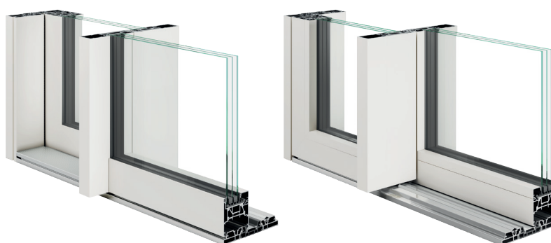
Scorrevole ASE 80 HI (vista interna ed esterna)
